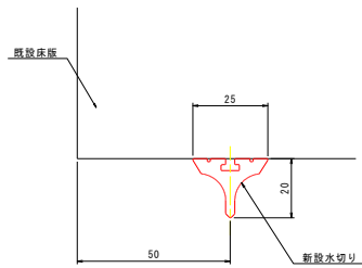
側面図
