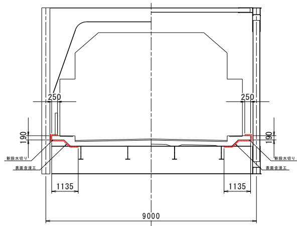
水切り詳細図 S=1:1
